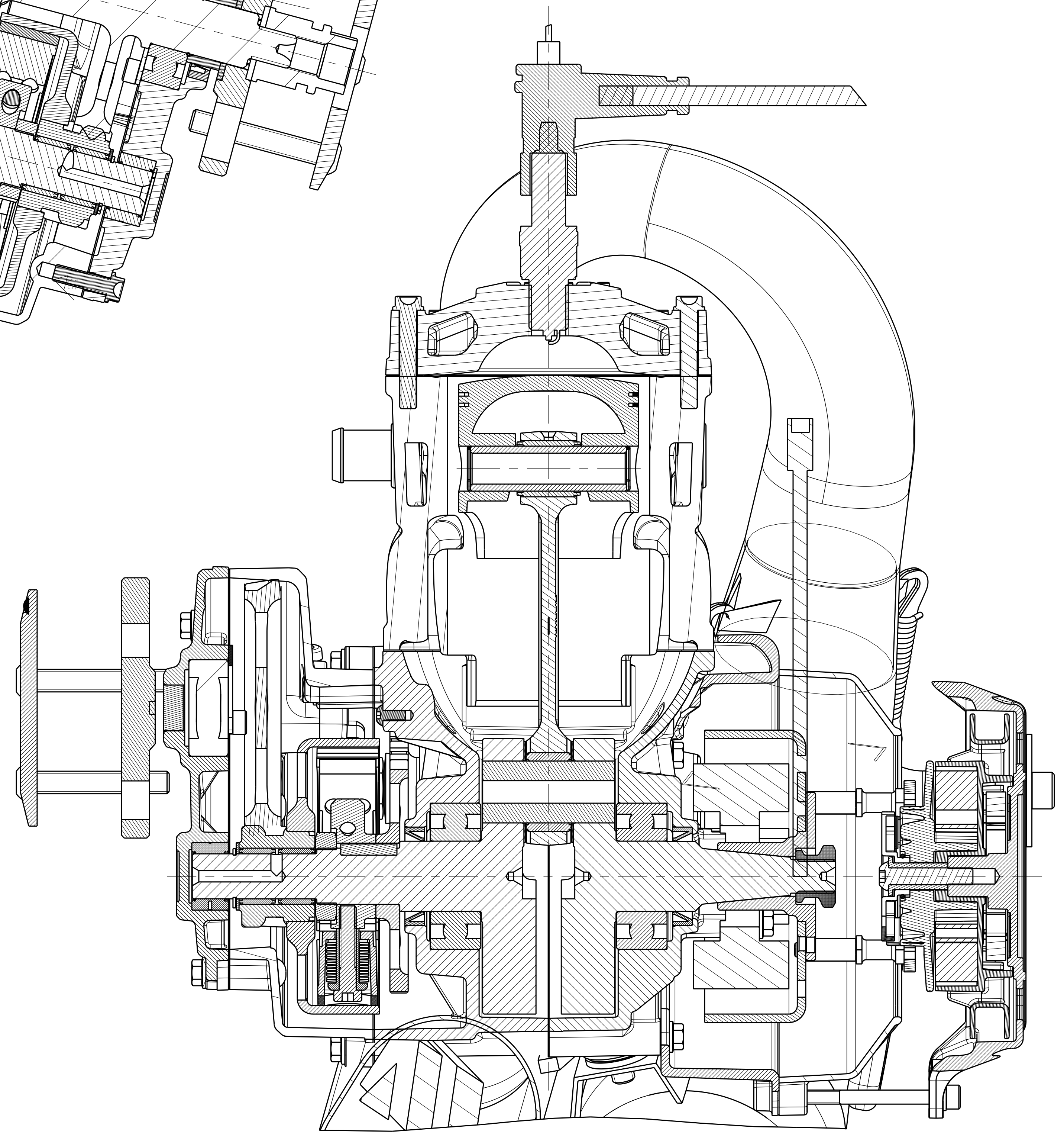
SEZIONE B-B
